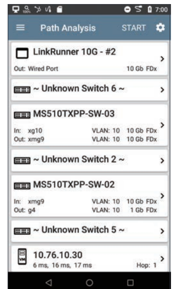
パス解析
